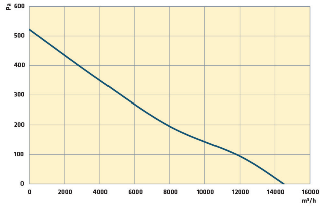
T/TAV 710-5-30 T4 1,50 kW
