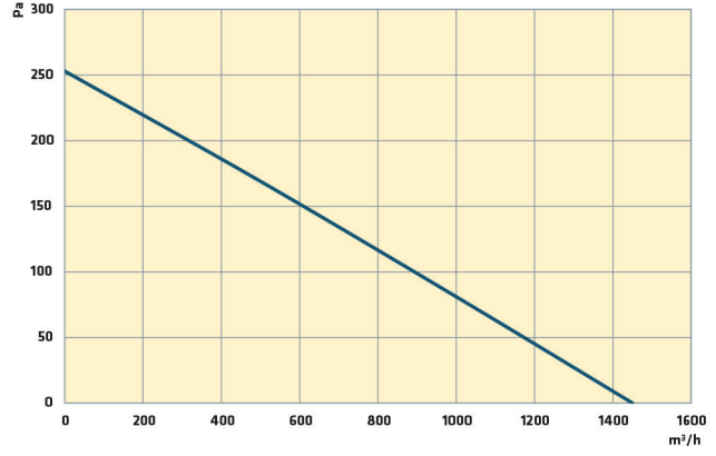
T/TAV 450-5-25 T4 0,55 kW
