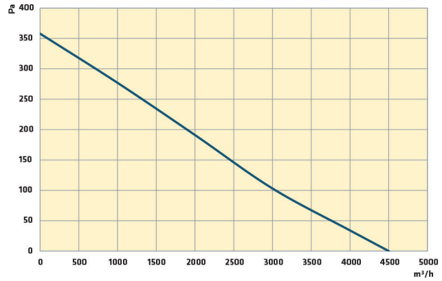
T/TAV 560-5-25 T4 0,75 kW
