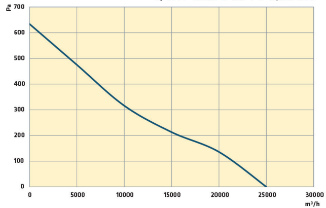
T/TAV 800-5-35 T4 3,00 kW
