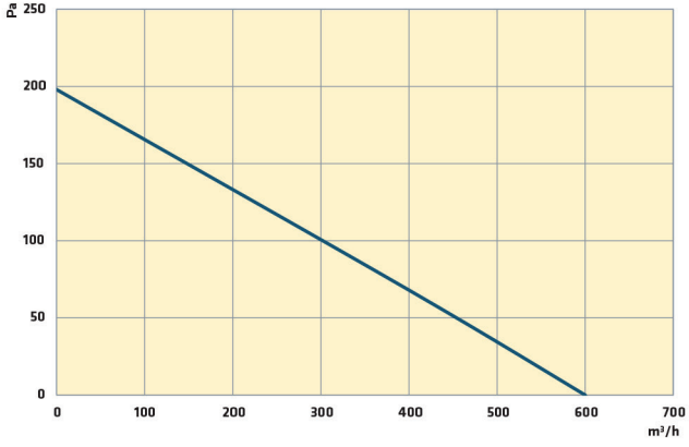
T/TAV 400-5-25 T4 0,37 kW
