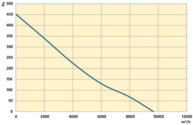
T/TAV 630-5-30 T4 1,10 kW
