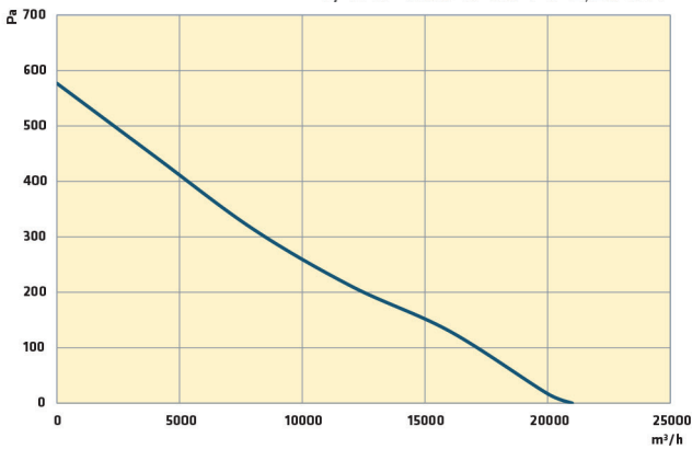
T/TAV 800-5-30 T4 2,20 kW
