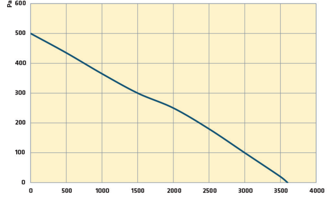
T/AXB-F 900x650 M4 0,9 kW
