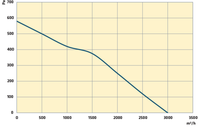
T/AXB-F 900x650 M4 0,64 kW
